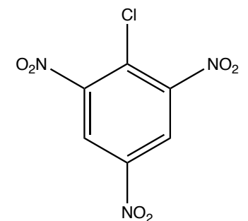
2-chloro-1,3,5-trinitrobenzene
