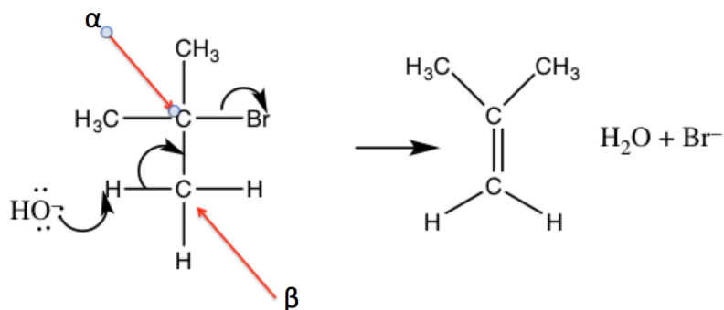
An E2 Elimination
