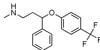
Prozac
